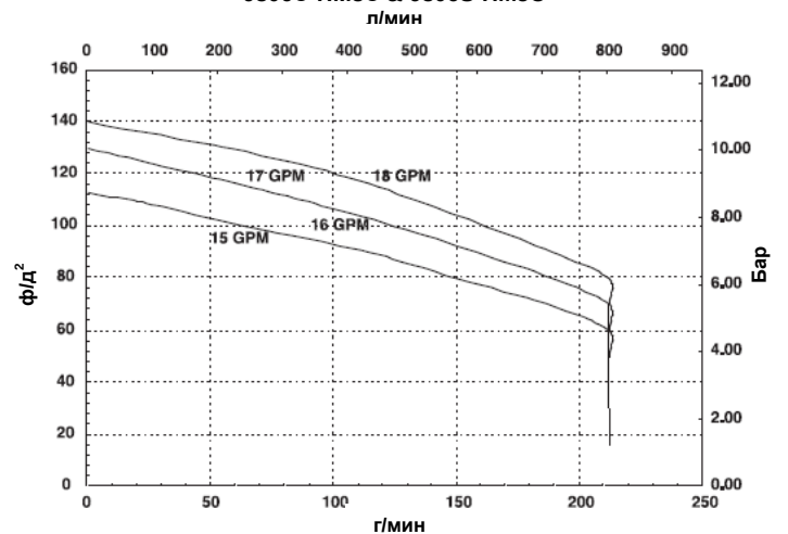
9306C-HM5C & 9306S-HM5C
